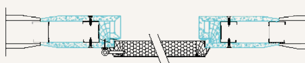
Coupe horizontale, système à recouvrement
